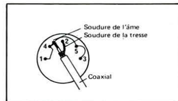
FIGURE 2: Câblage de la prise «vidéo»
