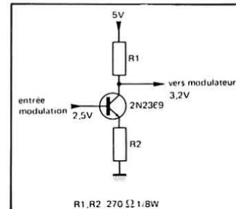
FIGURE 5: Schéma de l'inverseur de modulation
