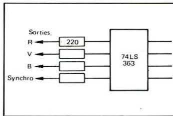
FIGURE 1: Sortie RVB de l'ORIC
