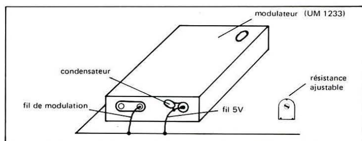
FIGURE 6: Vue de l'implantation sur le circuit imprimé
