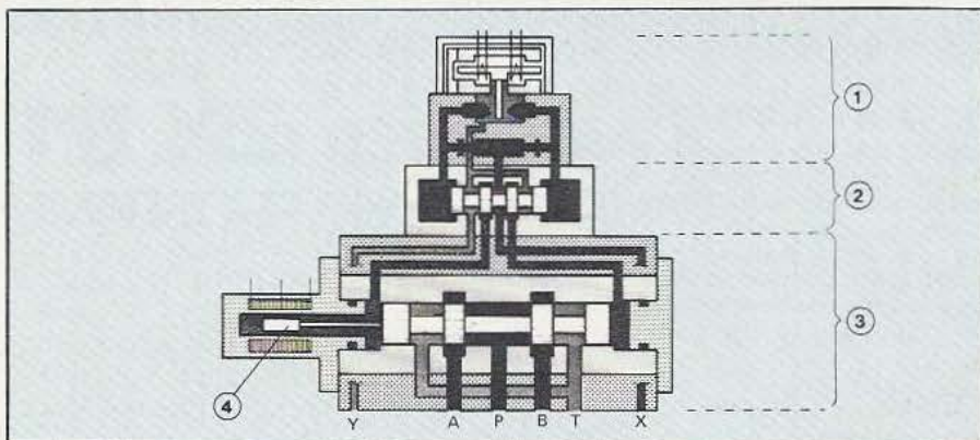
Les 3 étages d'une servo-valve à contre-réaction électrique (4).
