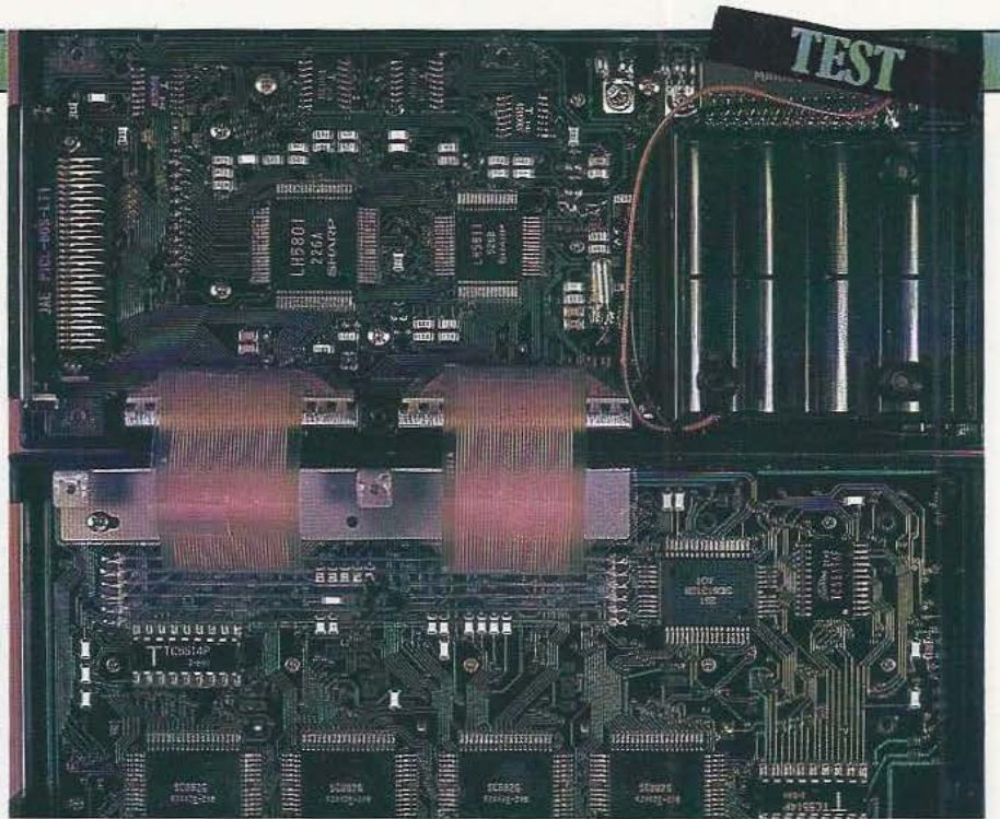
Un double circuit imprimé regroupant de nombreux circuits intégrés «flat pack».
