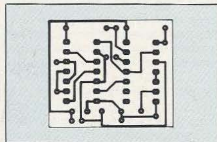
Fig. 6. Circuit imprimé côté cuivre.
