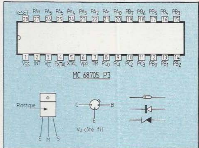
Fig. 9. Brochages du 68705 P3, des semi-conducteurs...
