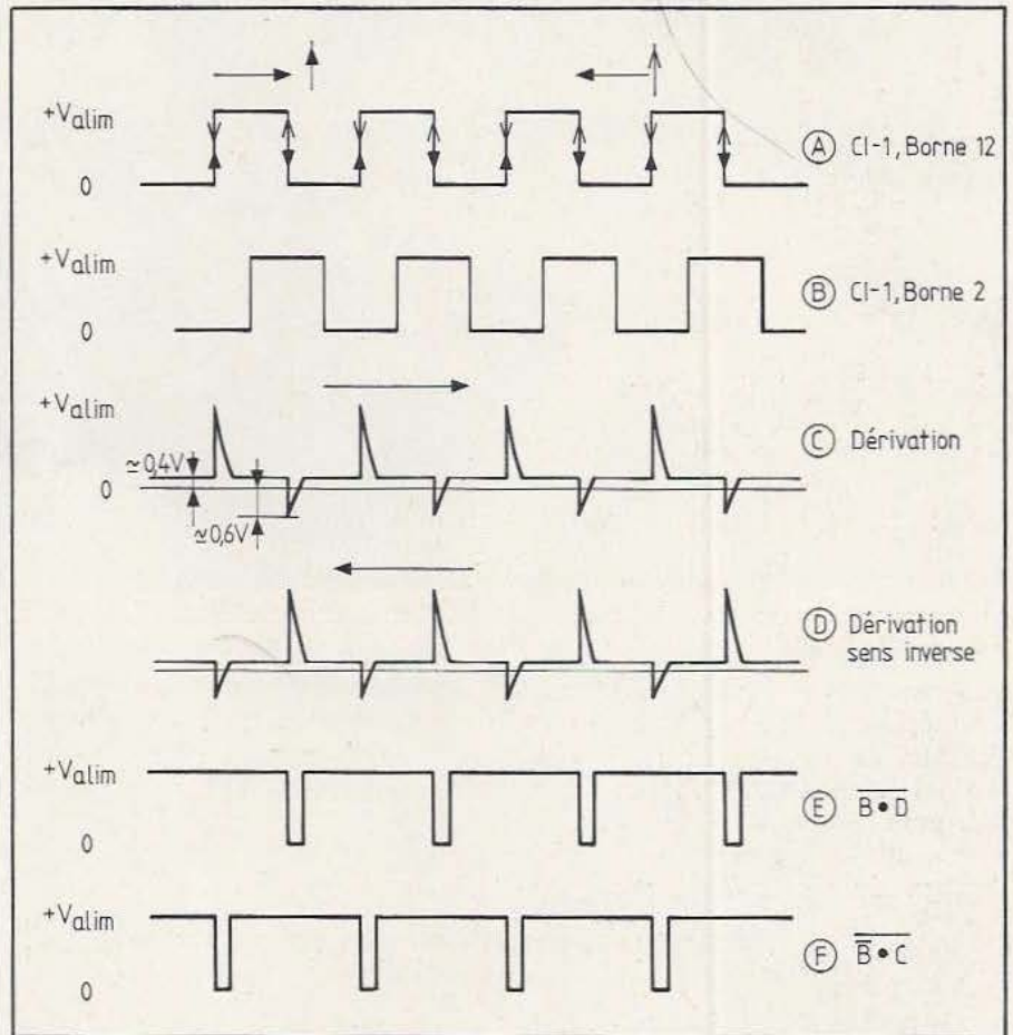
Fig. 4. Forme des signaux recueillis à différents points du circuit.
