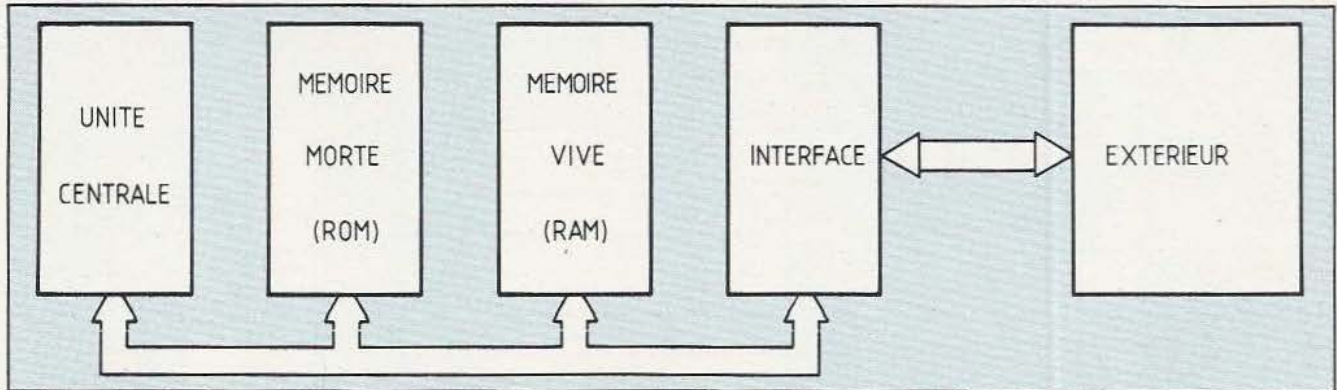
Fig. 1 : Synoptique de tout micro-ordinateur : UAL, ROM, RAM et interface.
