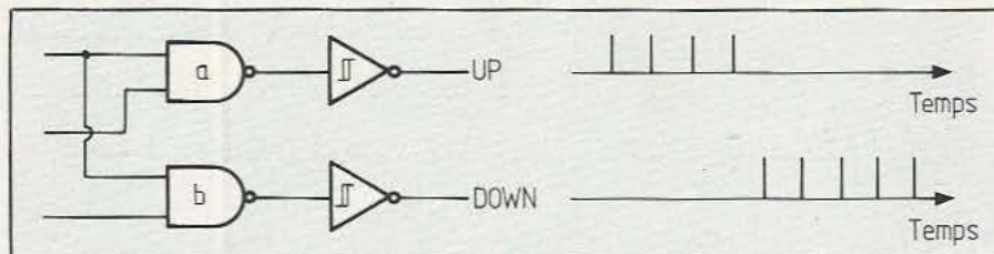
Fig. 5. Génération de trains d'impulsions selon le sens de rotation.
