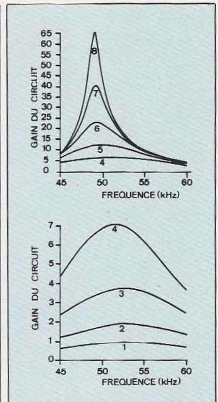
Fig. 3. En haut, réponses typiques du passe-bande en fonction du paramètre distance (ordonnées en dB). En bas réponses amplitude/fréquence de l'amplificateur de contrôle.
