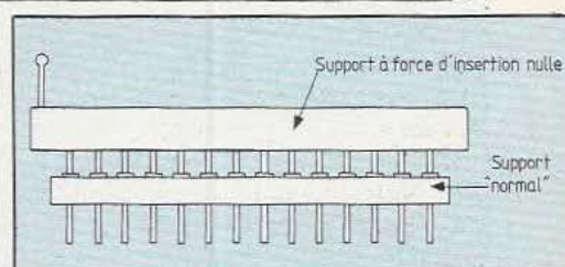
Fig. 5. Mise en place des 2 supports.
