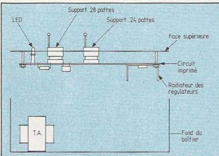
Fig. 8. Mise en place dans le coffret.
