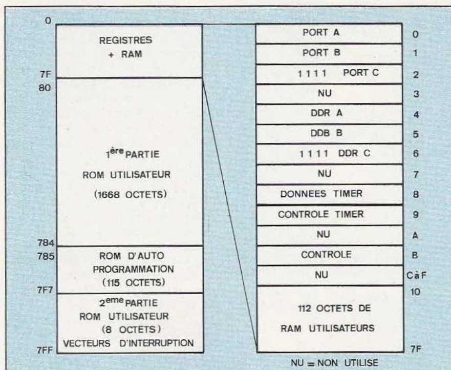
Fig. 4 : Organisation mémoire du 68705 P3.
