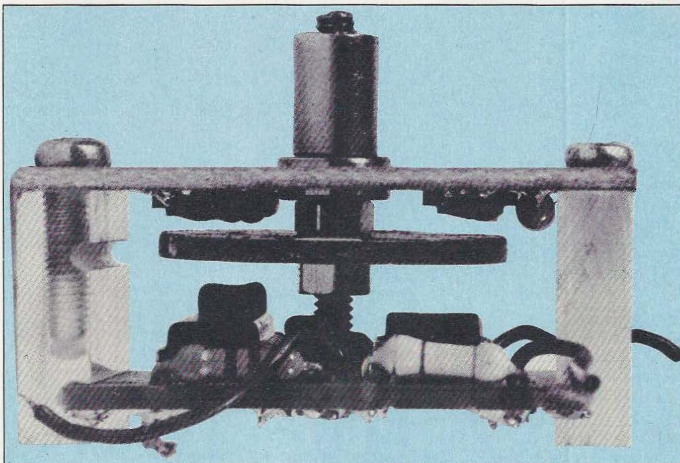
Le circuit imprimé principal (en bas) et la plaquette support des photo-coupleurs (en haut); largeur totale : 41 mm.
