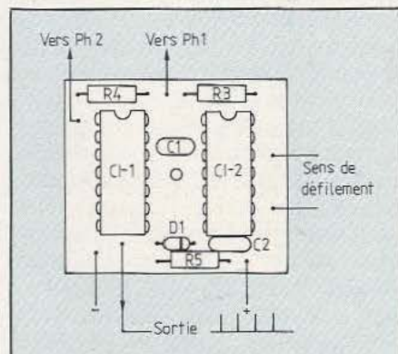
Fig. 7. Implantation des composants : R1 et R2 sont disposées à côté des détecteurs.
