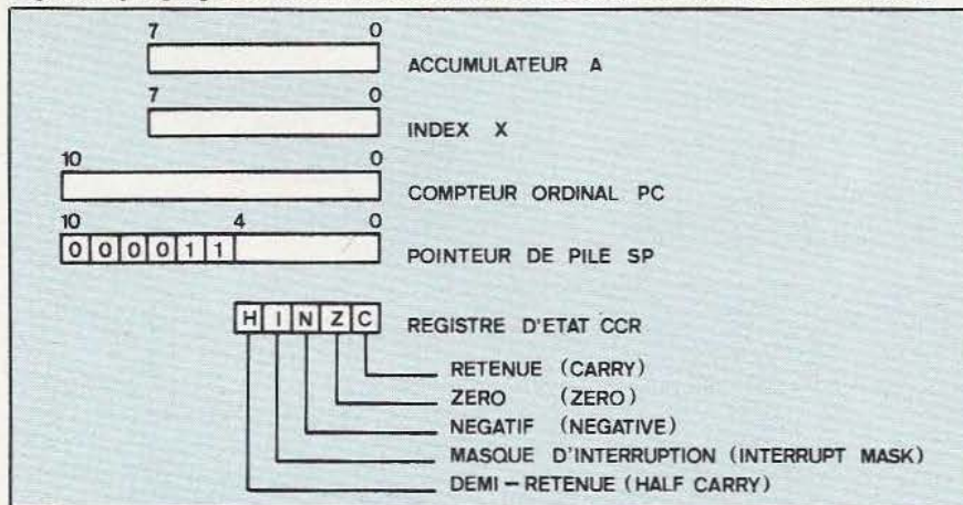
Fig. 2. Les registres internes du 68705 P3.
