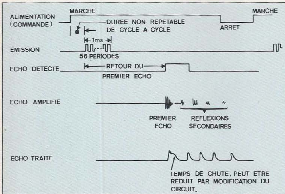
Fig. 4. Diagramme de fonctionnement du module émetteur-récepteur.
