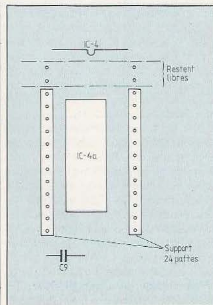
Fig. 4. Mise en place du support 24 pattes.
