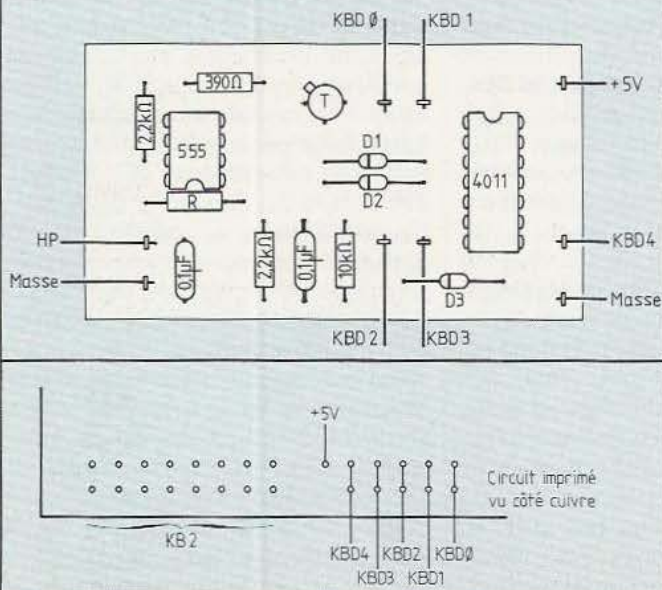
Fig. 9. Implantation des composants.
