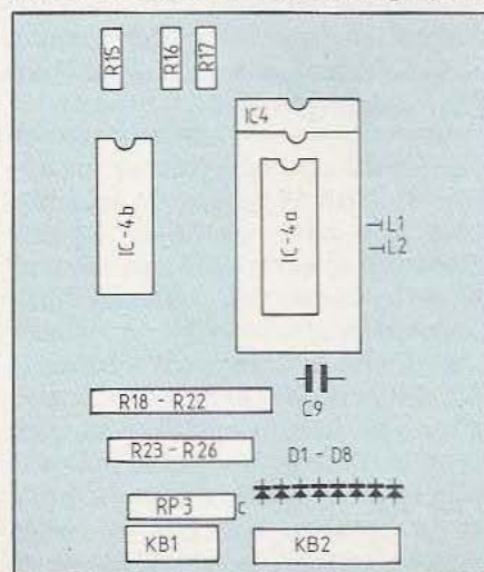
Fig. 3 Emplacement de la Ram interne.
