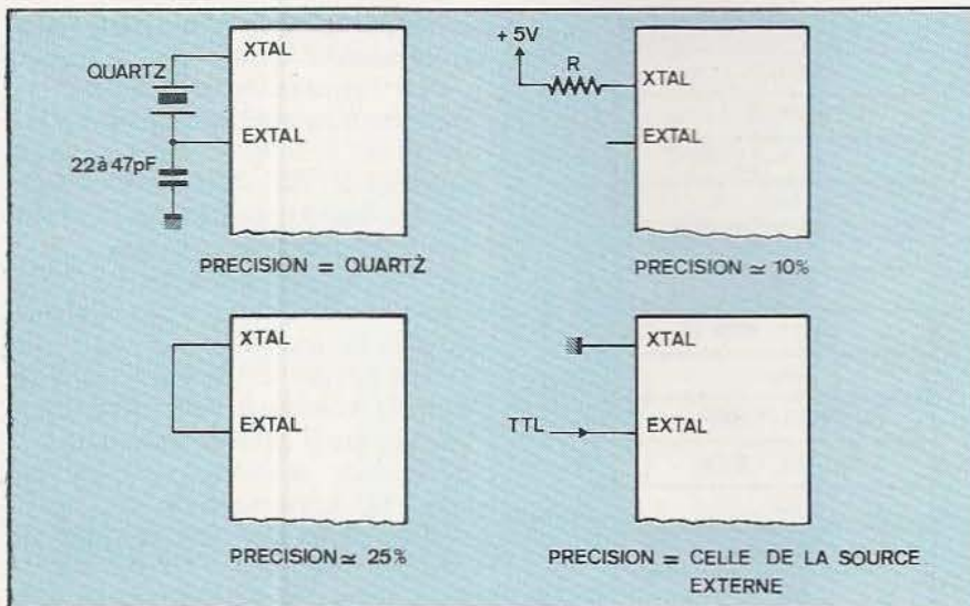
Fig. 5. Les quatre modes de génération d'horloge.
