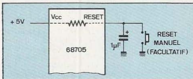
Fig. 6. Utilisation de l'entrée Reset.
