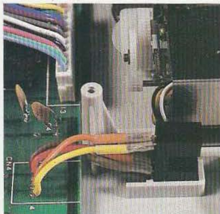
Détecteur optique de fin de papier.
