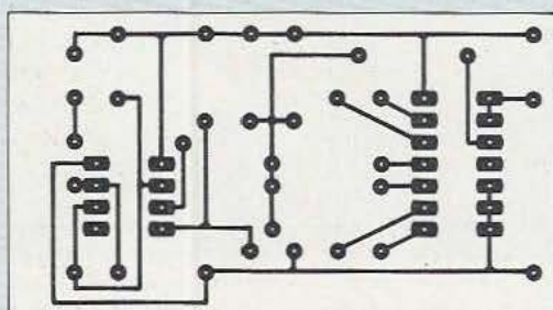
Fig. 8. Circuit imprimé, côté cuivre, échelle 1.
