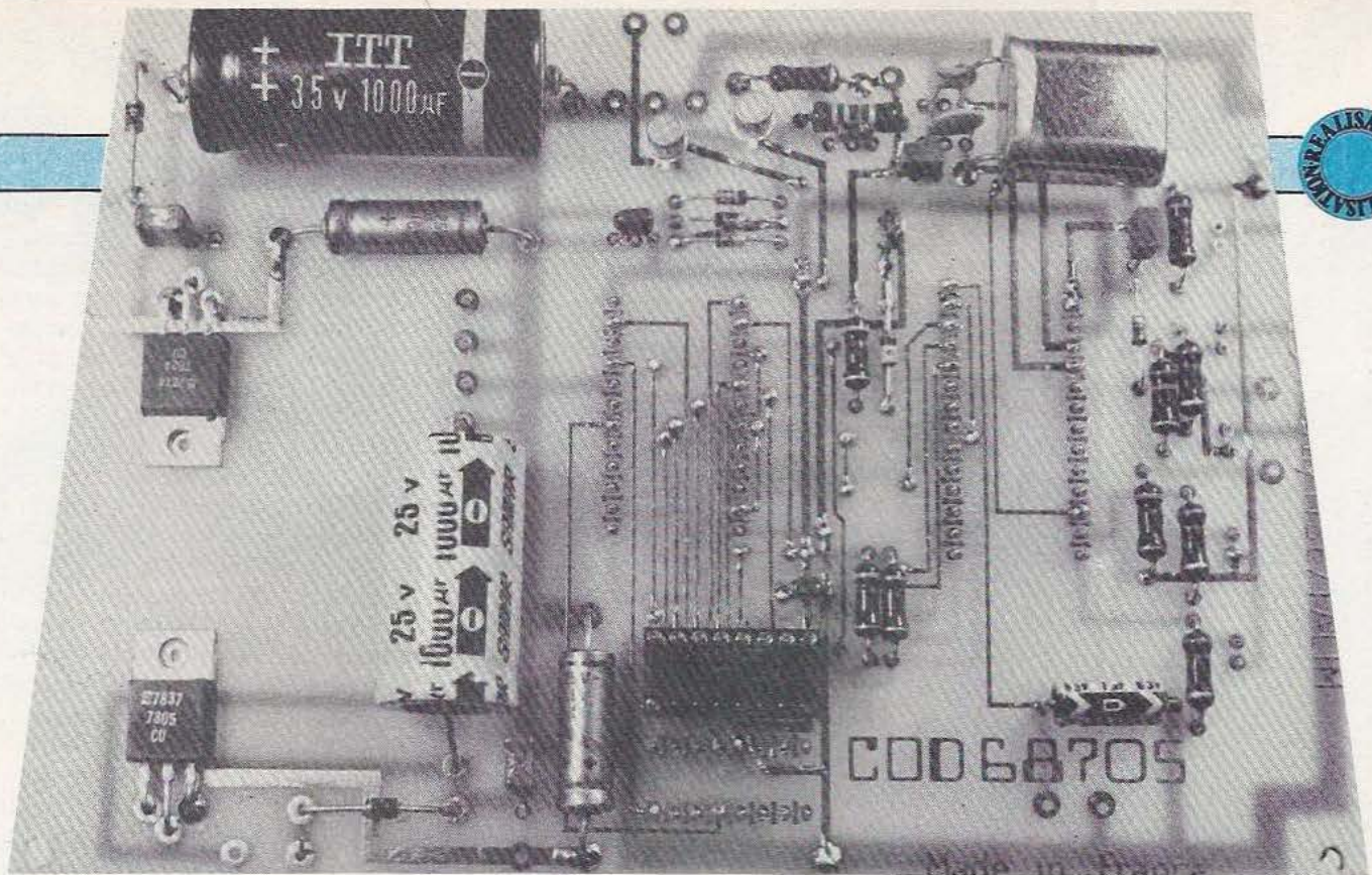
On s'aidera de cette photo pour l'implantation. Bien positionner les transistors et les régulateurs.
