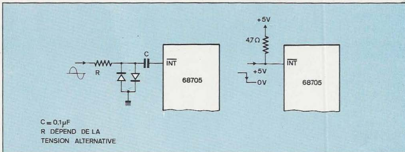
Fig. 7. Les deux possibilités d'emploi de l'entrée d'interruption.
