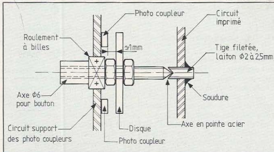
Fig. 8. Disposition mécanique des éléments, vue en coupe.
