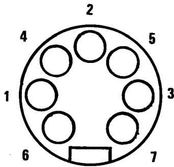
BROCHE VUE COTE SOUDURE
