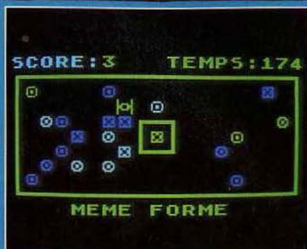
Chaos
