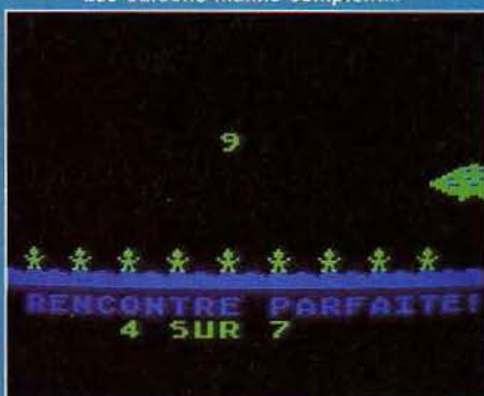
Extra-terrestres
