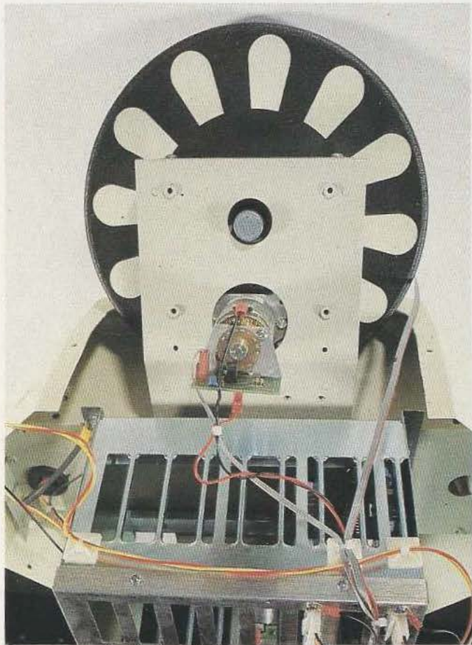
L'un des deux moteurs et son codeur incrémental.
