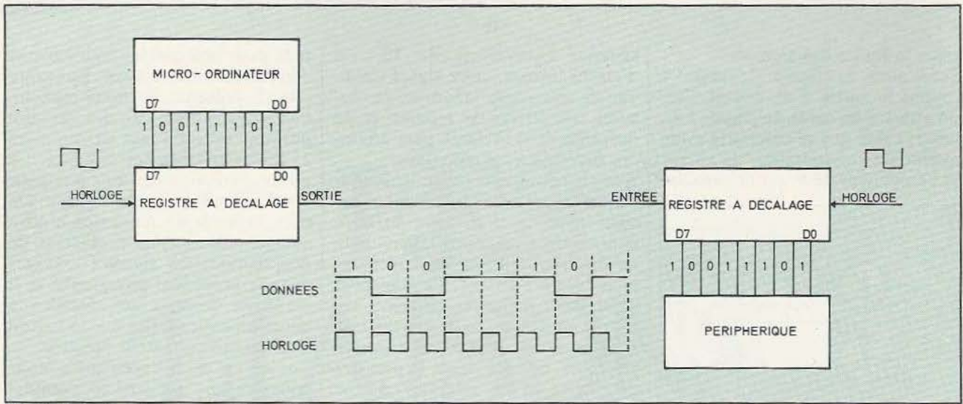
Fig. 2. Principe d'une transmission série.
