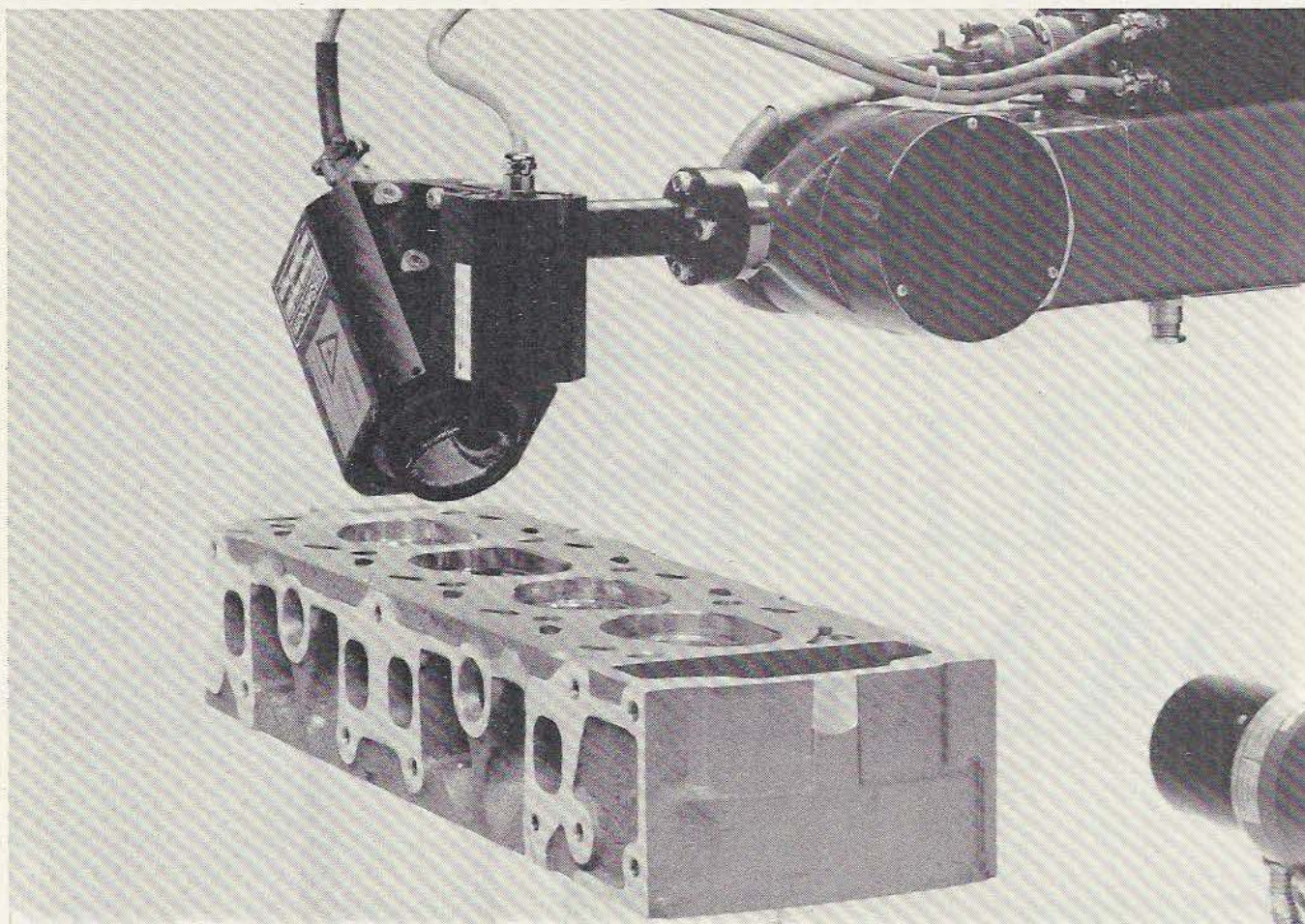
Le IRB 6, best-seller d'Asea en 83, fait ici du contrôle dimensionnel de pièces.
