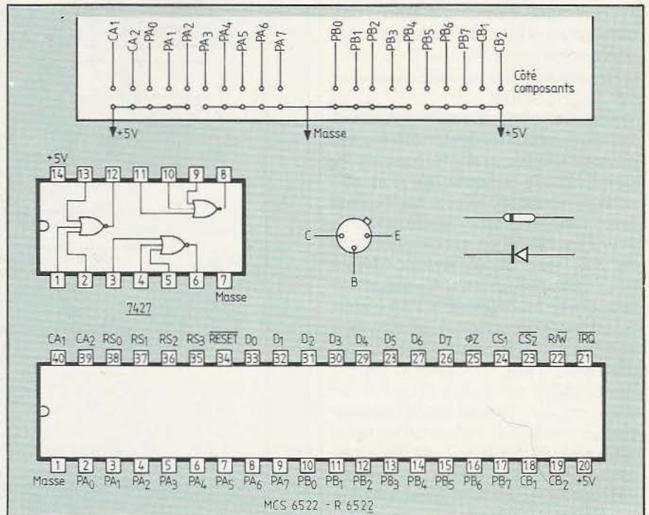
Fig. 7. Brochages et connexions.
