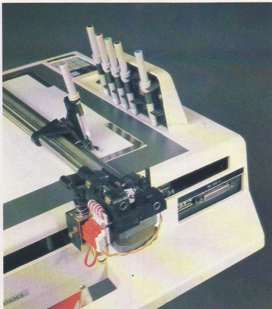
Remarquez les languettes magnétiques de fixation du papier.
