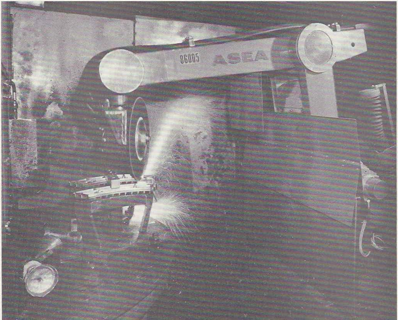
Le robot IRB 60 d'Asea «in situ» : le tronçonnage de jets de coulée.
