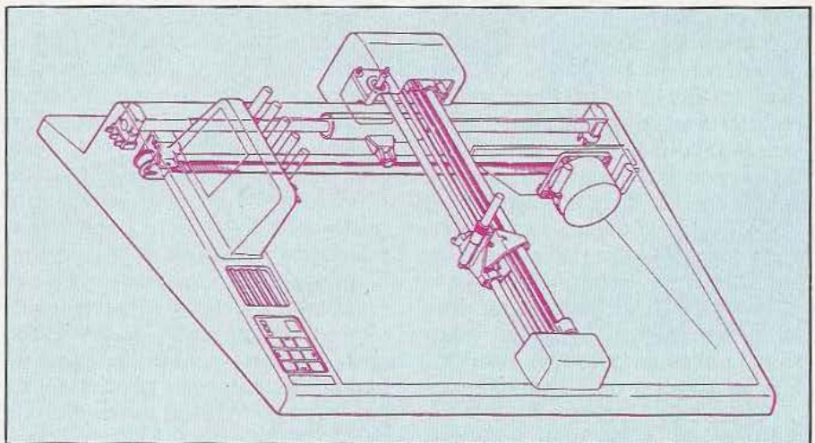
Figure 1 : éclaté de la table XY Graphtec.
