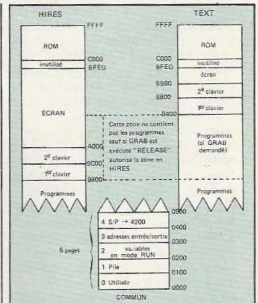
Fig. 2. Cartographie mémoire de l'Oric
