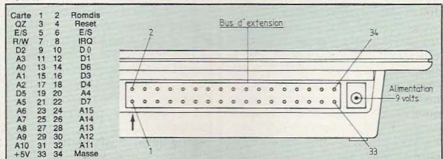
Fig. 6. Connecteur arrière de l'Oric.
