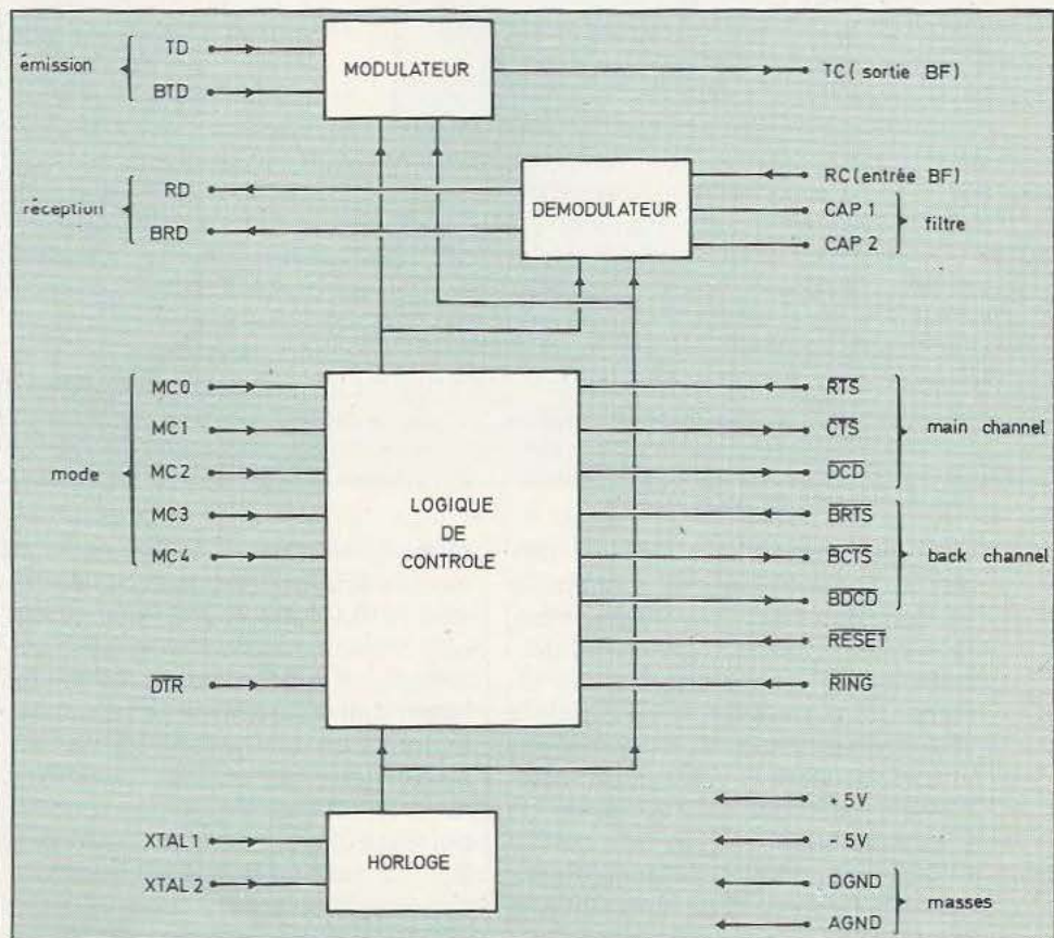
Fig. 9. Synoptique interne du modem intégré 7910.
