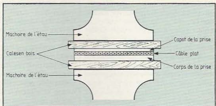
Fig. 5. Une méthode rapide de sertissage.
