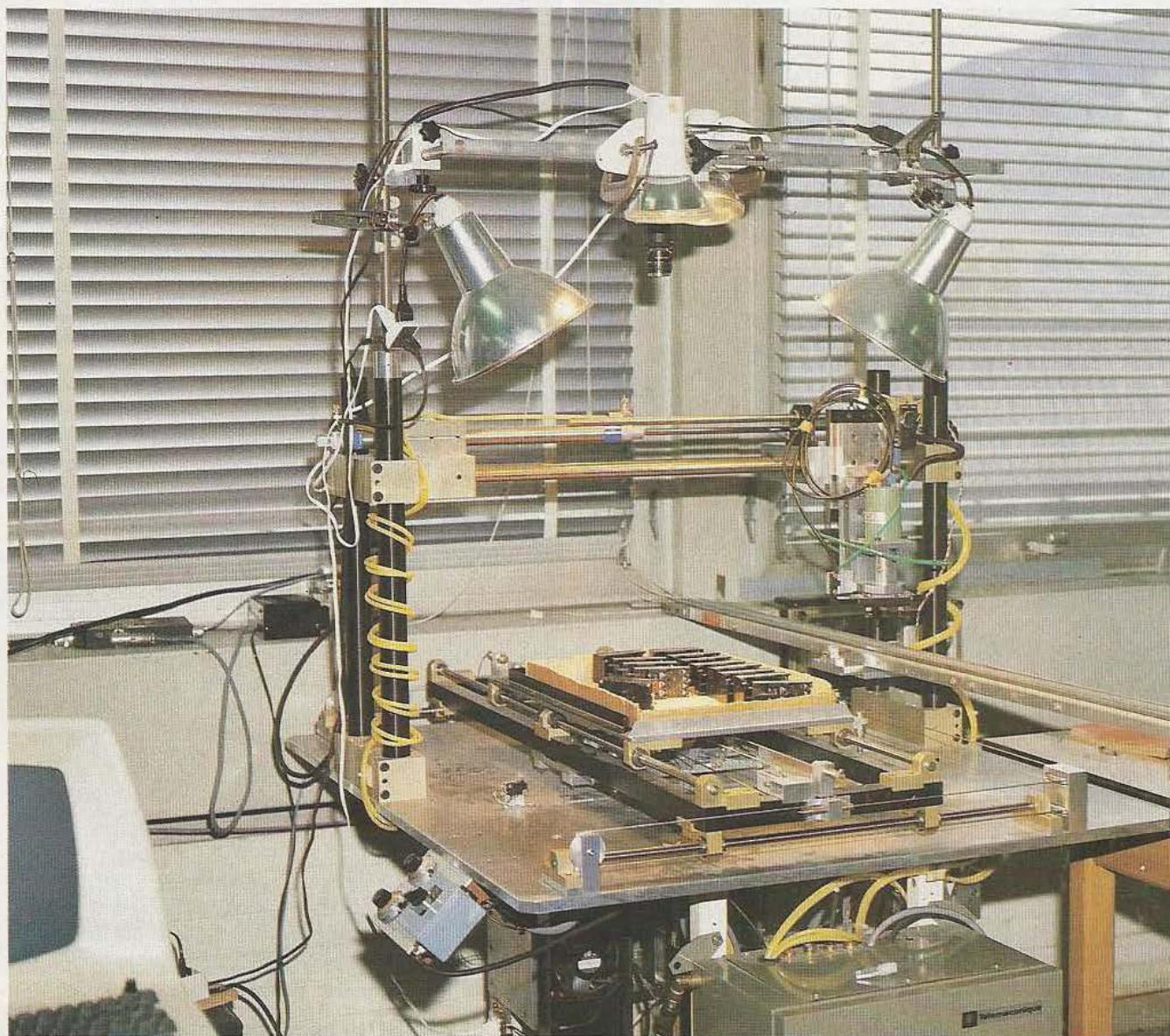
Reconnaissance de formes mise en pratique dans une «station de déchargement» de relais. Ceux-ci, placés dans un bac sont reconnus et saisis même s'ils sont mal orientés. Pour le moment le système ne traite que d'une seule phase d'équilibre.
