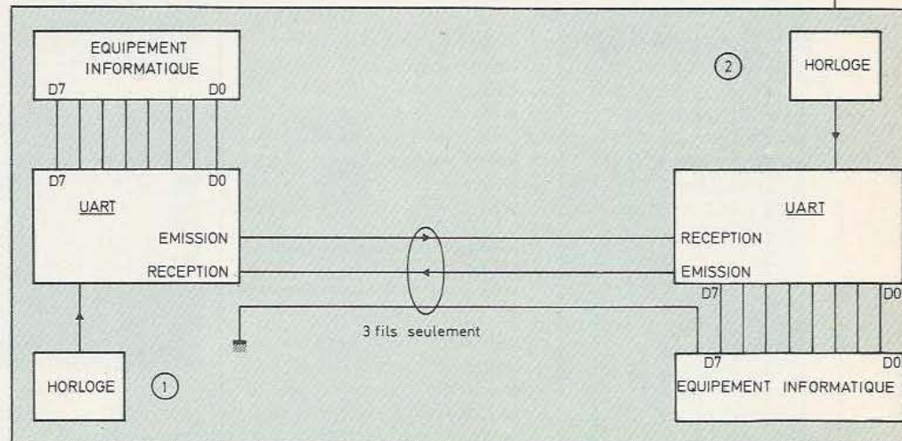
Fig. 5. Une liaison série asynchrone typique.
