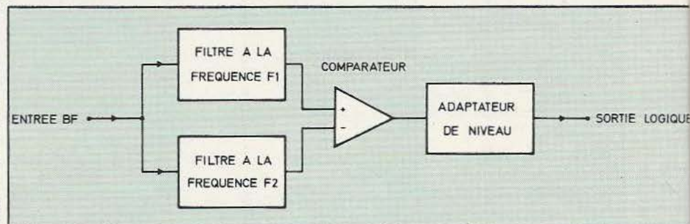
Fig. 4. Démodulateur à filtres.
