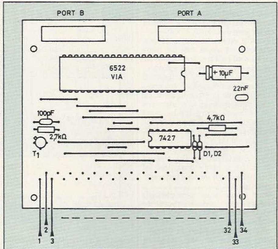
Fig. 4. Implantation des composants sur la carte.
