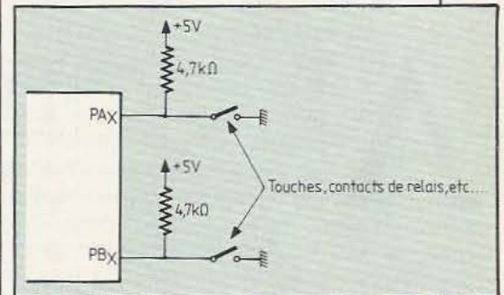
Fig. 11. Interfaçage de contacts.
