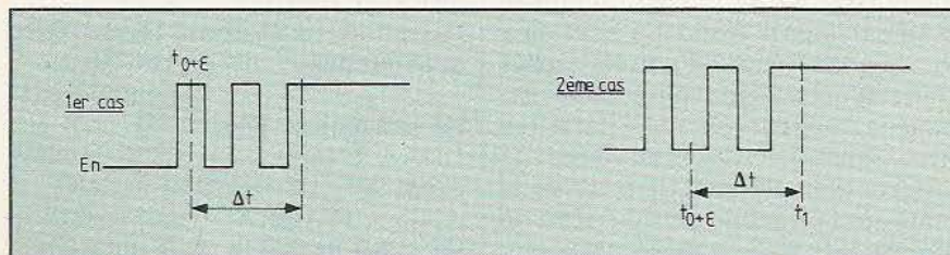
Figure 2. a) On mémorise E_n = 1 à t_0 + \epsilon ; on compare, au bout de \Delta t : E_n : 1 = E_n(\Delta t) = E_n(t_0 + \epsilon) , d'où E_n = 1 . b) On mémorise E_n = 0 à t_0 + \epsilon ; on compare à E_n au bout de \Delta t : E_n(\Delta t) \neq E_n(t_0 + \epsilon) ; donc on recommence. c) On mémorise E_n = 1 à l'instant t_1 ; on compare E_n du bout de \Delta t : E_n(\Delta t) = E_n(t_1) donc E_n = 1 . Le deuxième cas comporte la lecture d'un état transitoire : il faut donc, à nouveau, re-mémoriser et composer E_n .
