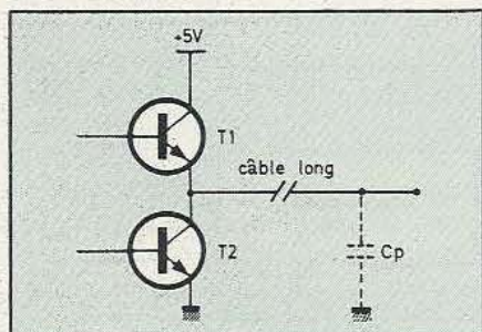
Fig. 1. Câble et capacité parasite.
