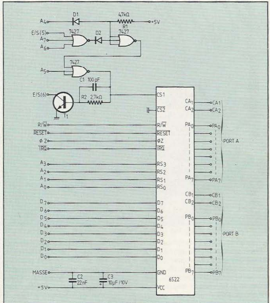
Fig. 1. Le schéma de principe retenu pour cette réalisation.
