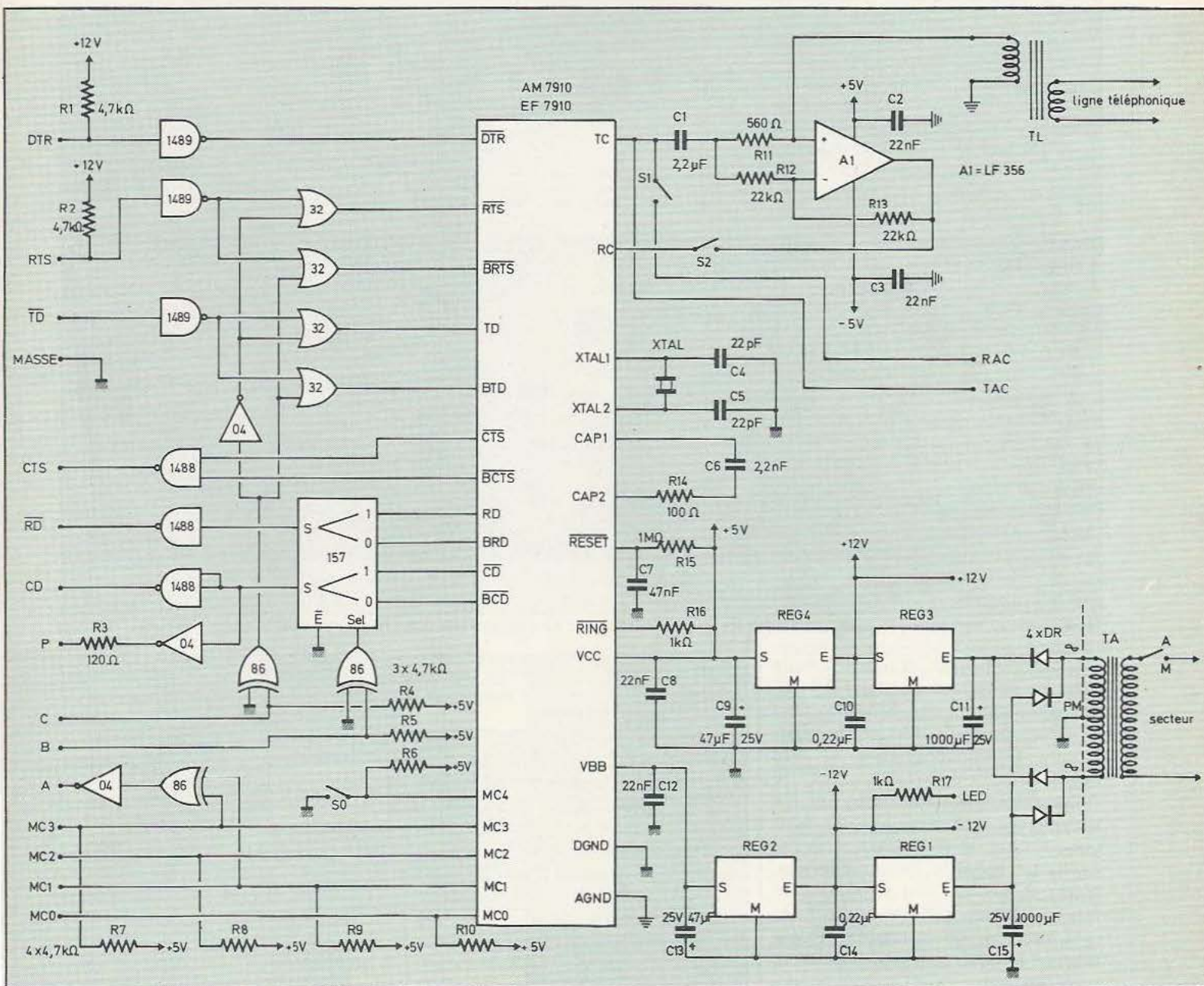
Fig. 8. Schéma de notre modem.
