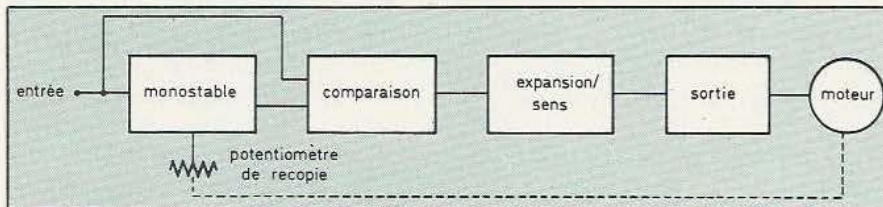
Fig. 2. Schéma synoptique d'un asservissement à circuit intégré.
