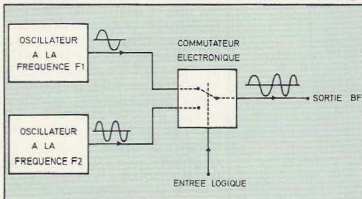
Fig. 2. Synoptique du modulateur d'un modem simple.
