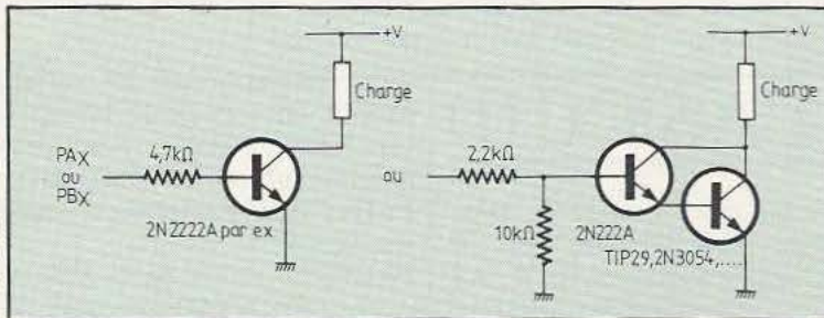
Fig. 8. Selon la charge on choisira un buffer à un transistor ou un Darlington.
