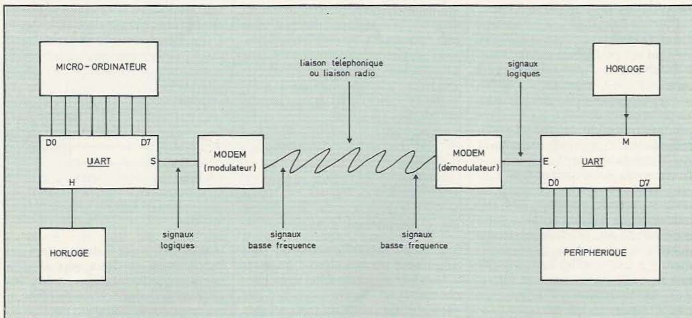
Fig. 1. La place d'un modem dans une liaison série.
