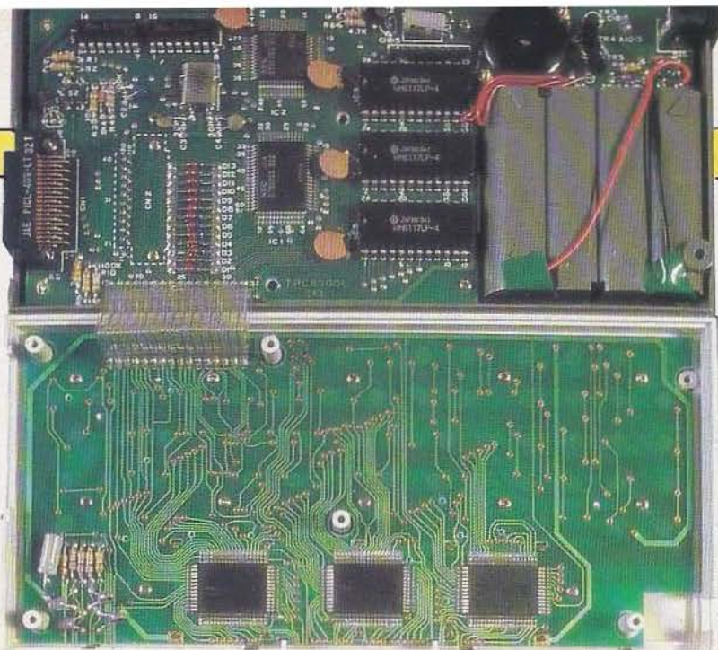
Le Sanco TPC 8300.. à cœur ouvert.
