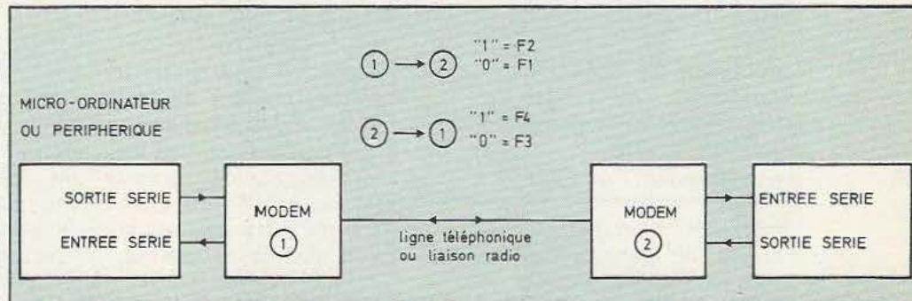
Fig. 6. Liaison bidirectionnelle par modem.
