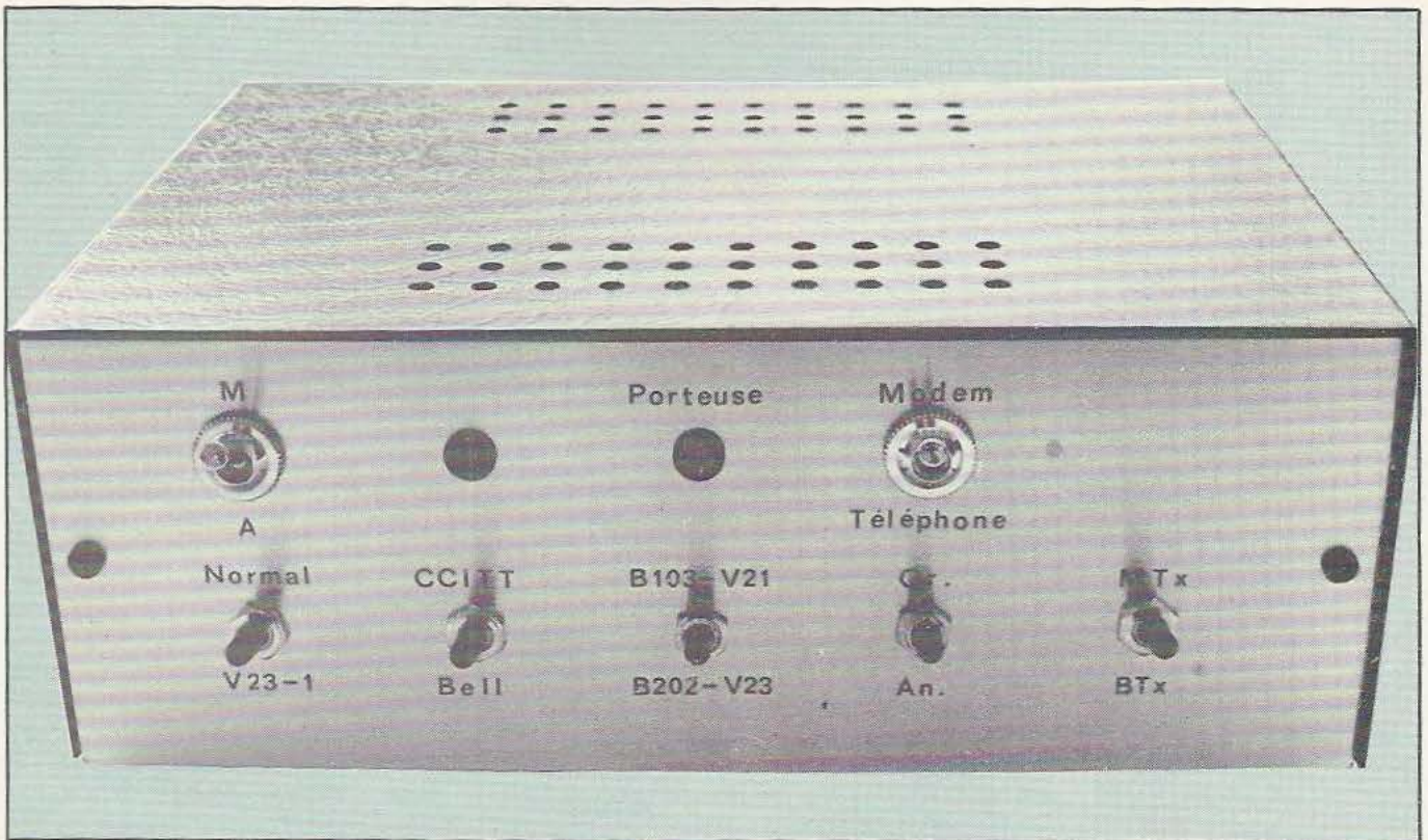
La face avant du coffret regroupant toutes les commandes: nous en reparlerons dans la seconde partie de cet article.
