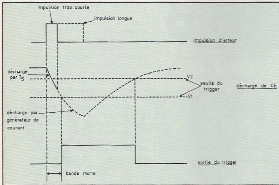
Fig. 4. Diagramme de fonctionnement du NE 544.
