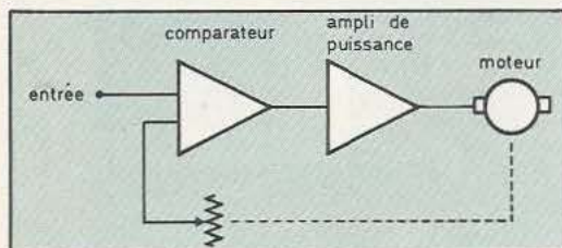
Fig. 1. Synoptique du schéma utilisé.
