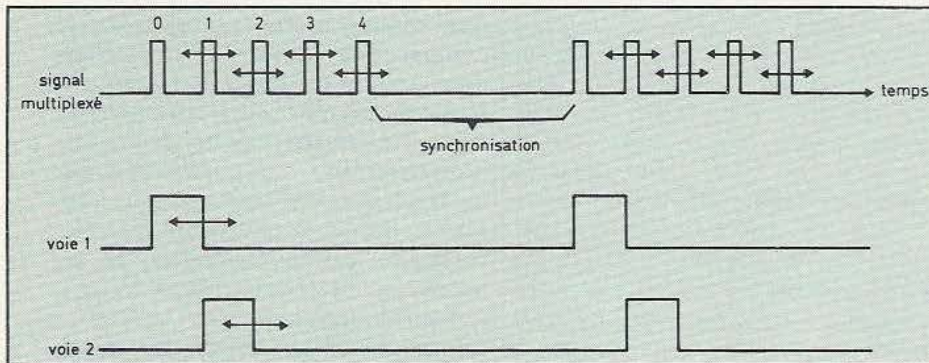
Fig. 1. Le principe : un train d'impulsions modulées en position.
