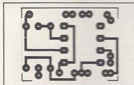
Fig. 4. Le circuit imprimé (éch. 2).
