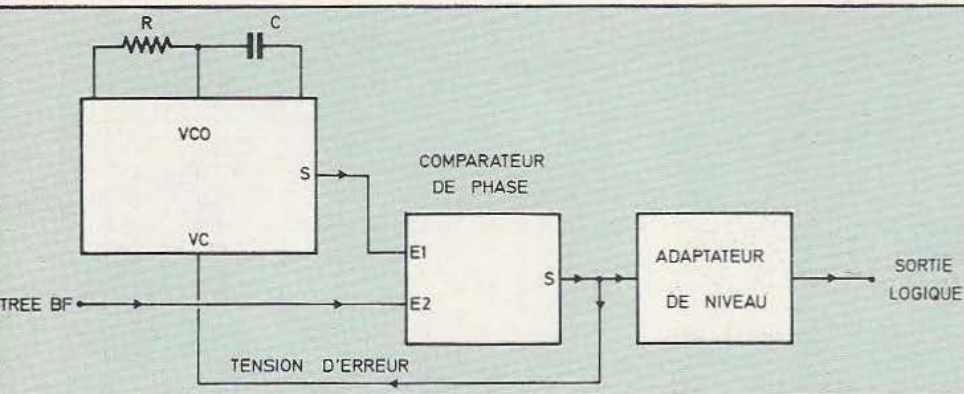
Fig. 5. Démodulateur à boucle à verrouillage de phase.
