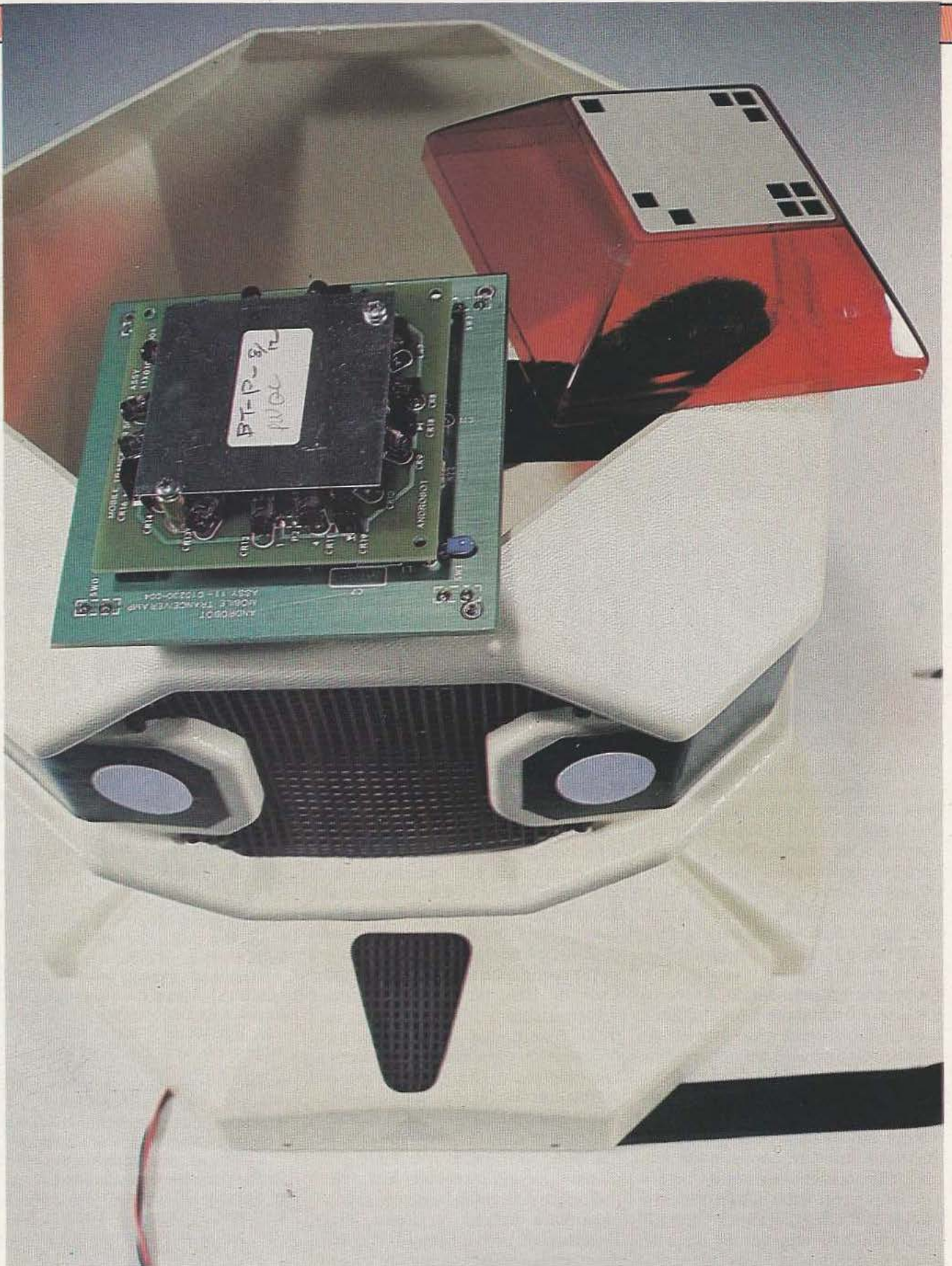
Une tête bien faite, plutôt que pleine : au sommet de son crâne le contacteur et le système infrarouge.
