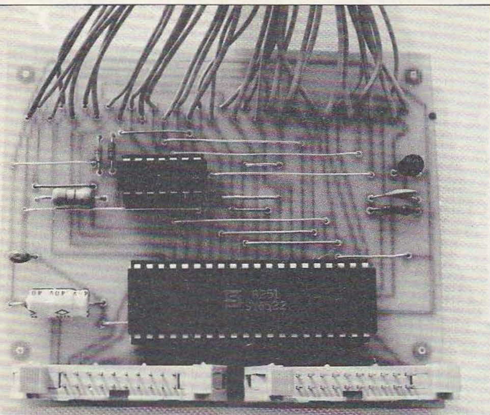
Le circuit imprimé simple face (d'où les straps...).
