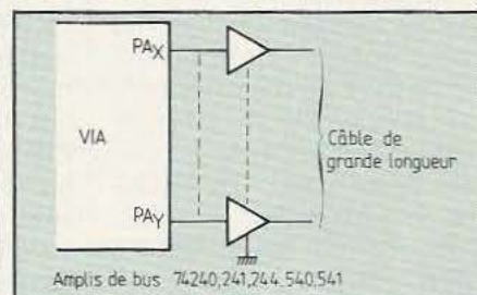
Fig. 9. Câbles longs:boostage nécessaire.
