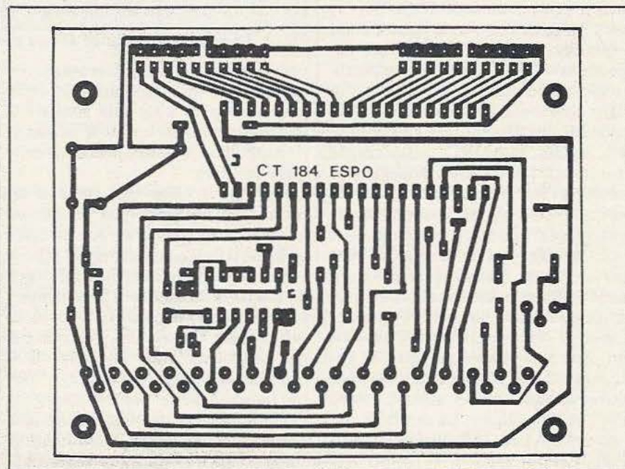
Fig. 3. Vue du circuit imprimé côté cuivre (échelle 1).
