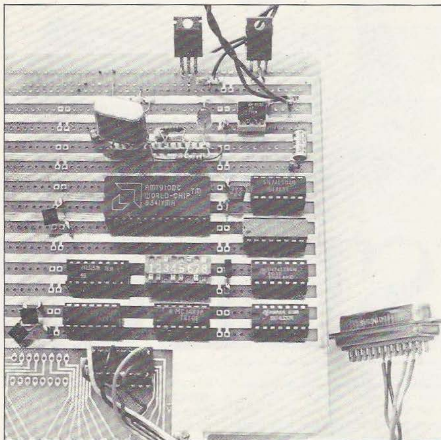
La carte qui a servi à mettre au point cette réalisation.
