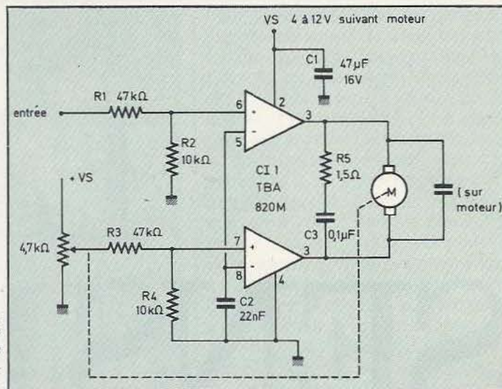
Fig. 2. Schéma de principe de l'asservissement proposé.
