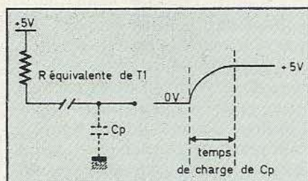
Influence sur le temps de montée.
