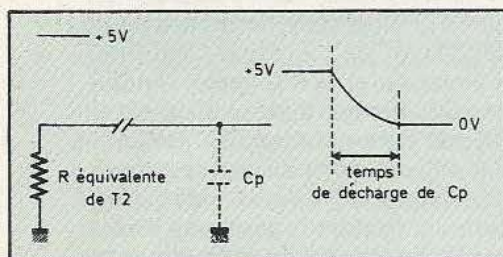
Dégradation du temps de descente.
