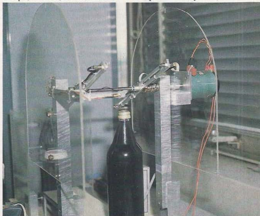
Passage entre deux capteurs en rotation d'un objet à reconnaître.
