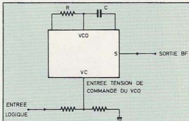
Fig. 3. Modulateur utilisant un VCO.
