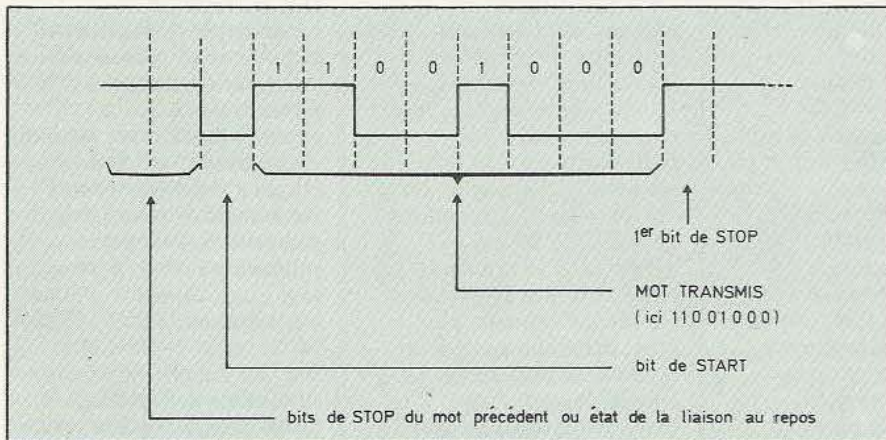
Fig. 4. Allure d'un caractère dans une transmission série synchrone.
