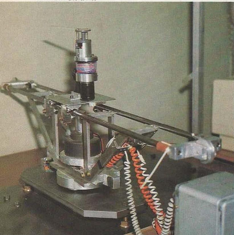
Expérience sur un actionneur plan à retour d'effort.
