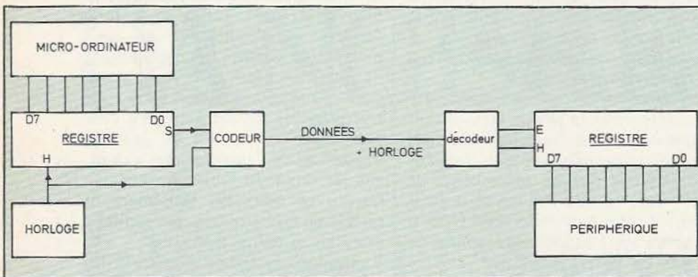
Fig. 3. Principe d'une liaison série synchrone.
