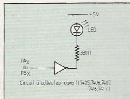
Fig. 10. Commande de Led.
