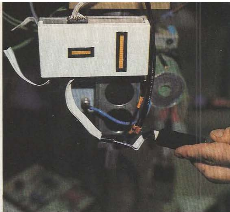
Peau sensible et traitement des signaux captés.
