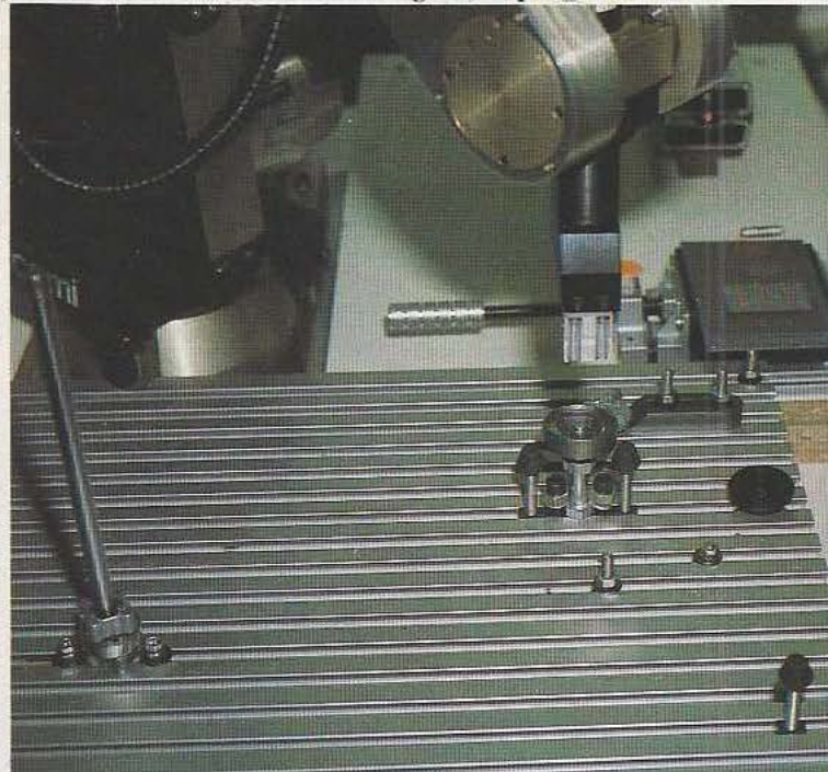
Montage d'un amortisseur à partir d'un robot Scemi.
